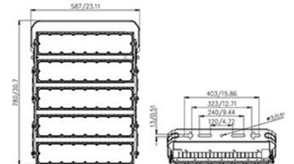
5 module 1200W
