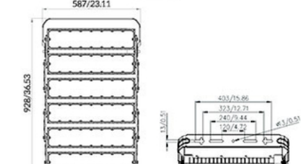
6 module 1440W
