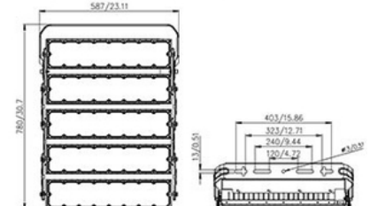
5 module 1200W
